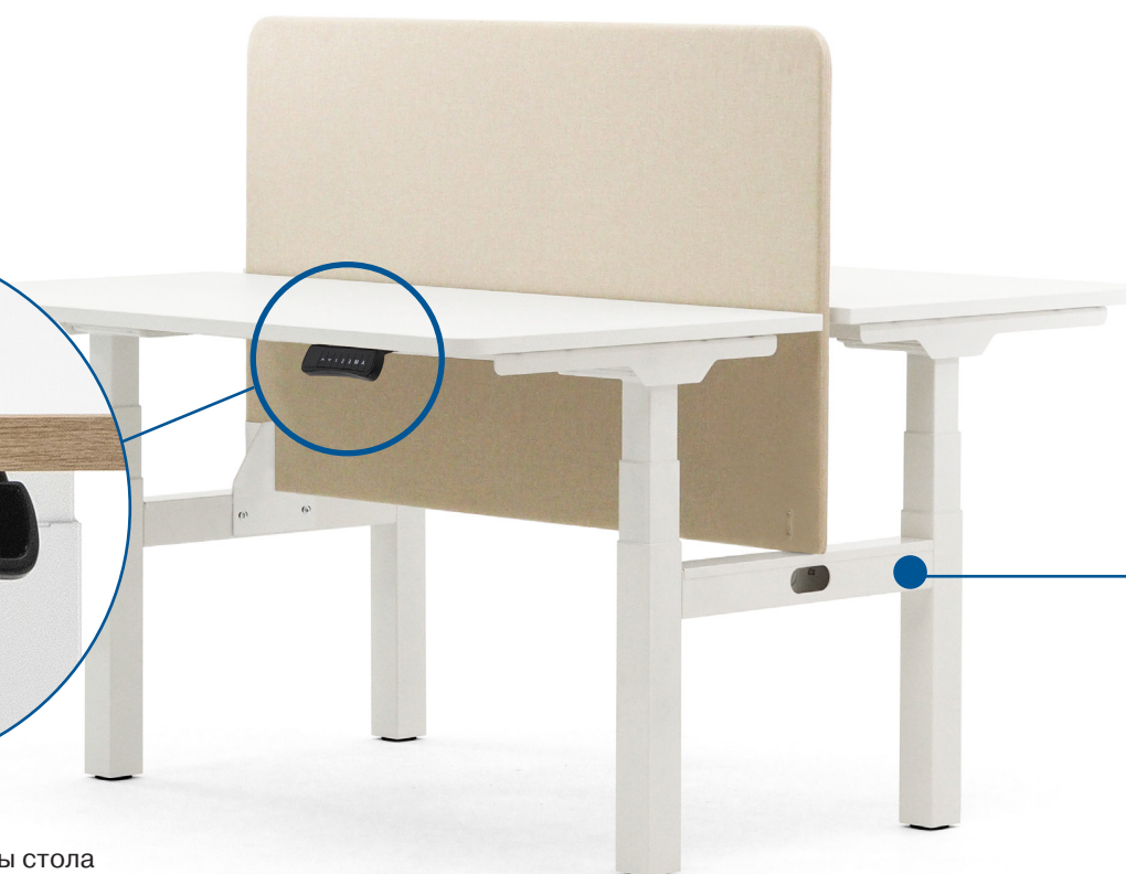
соединительная траверса со съемной крышкой для хранения и проводки кабелей
